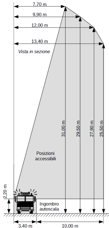
Illustrazione S.9-2: Sviluppo autoscala e posizioni accessibili
